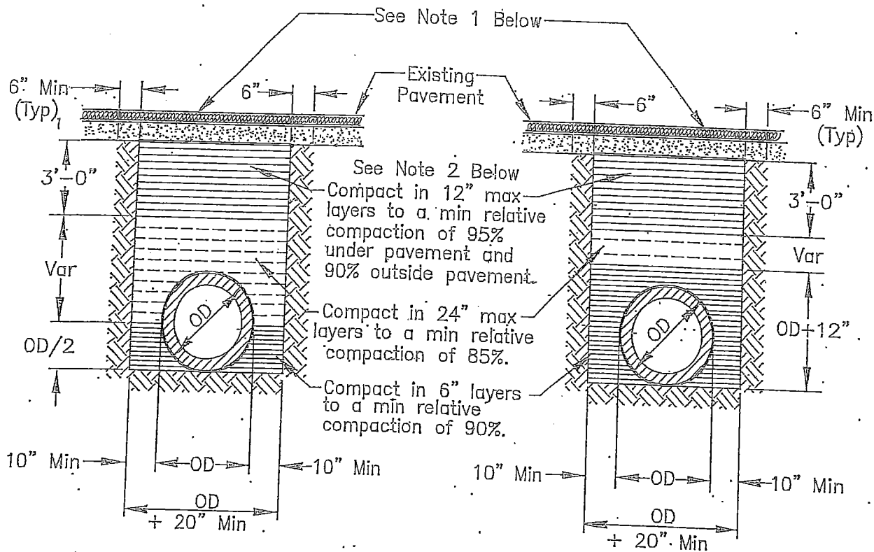
RIGID CONDUIT
